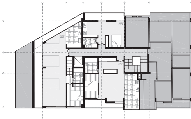
Piso 4 1_100
