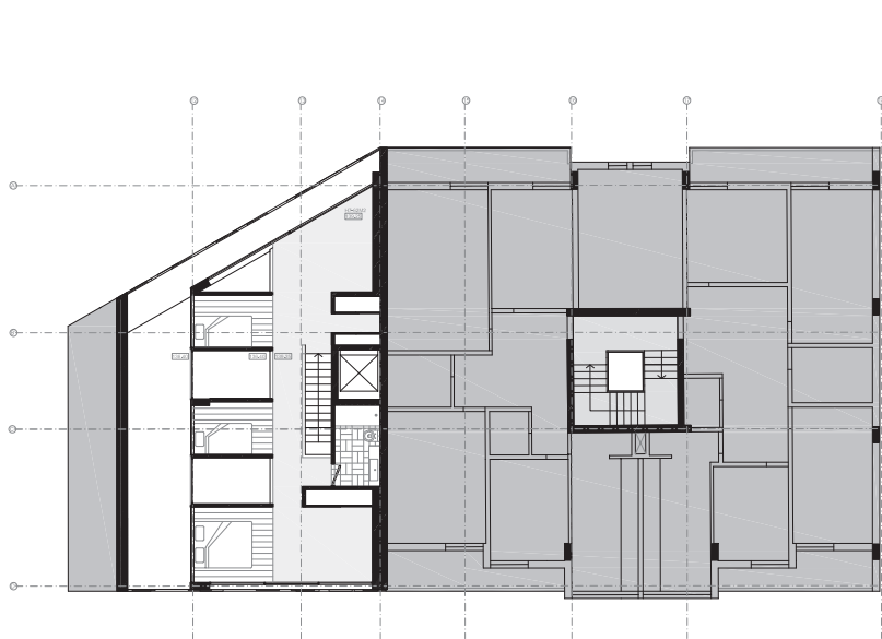
Piso 3 1_100
