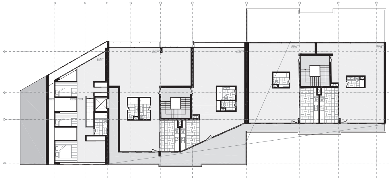
Piso 5 1_100
