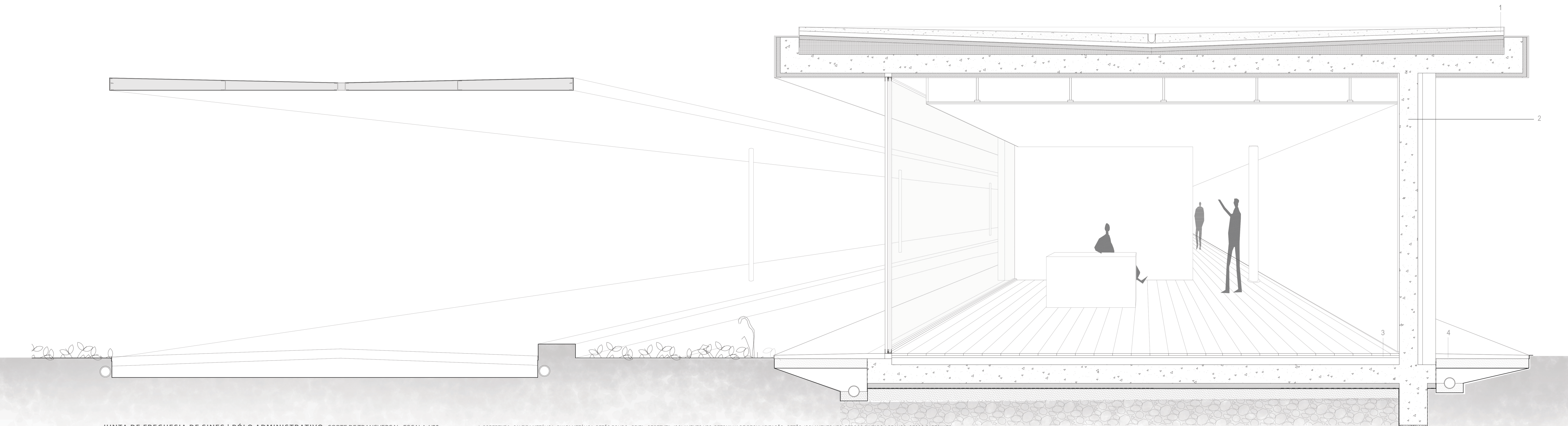
JUNTA DE FREGUESIA DE SINES | PÓLO ADMINISTRATIVO. CORTE DE TRANSVERSAL. ESCALA 1/20 PROJETO FINAL DE ARQUITETURA. ISCTE-IUL | DOCENTE: PEDRO PINTO .DISCENTE: ANDREIA M. TAVARES, OUTUBRO, 2016
