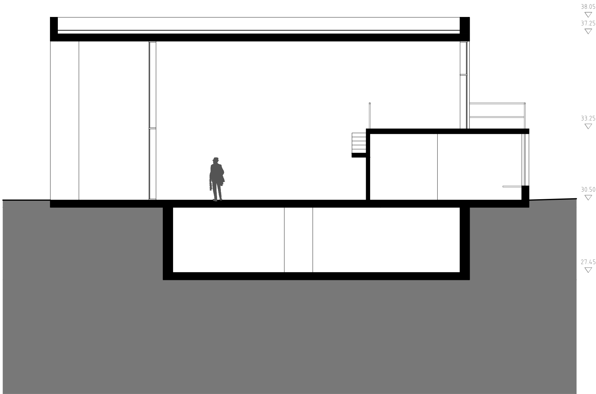
CORTE FF'
