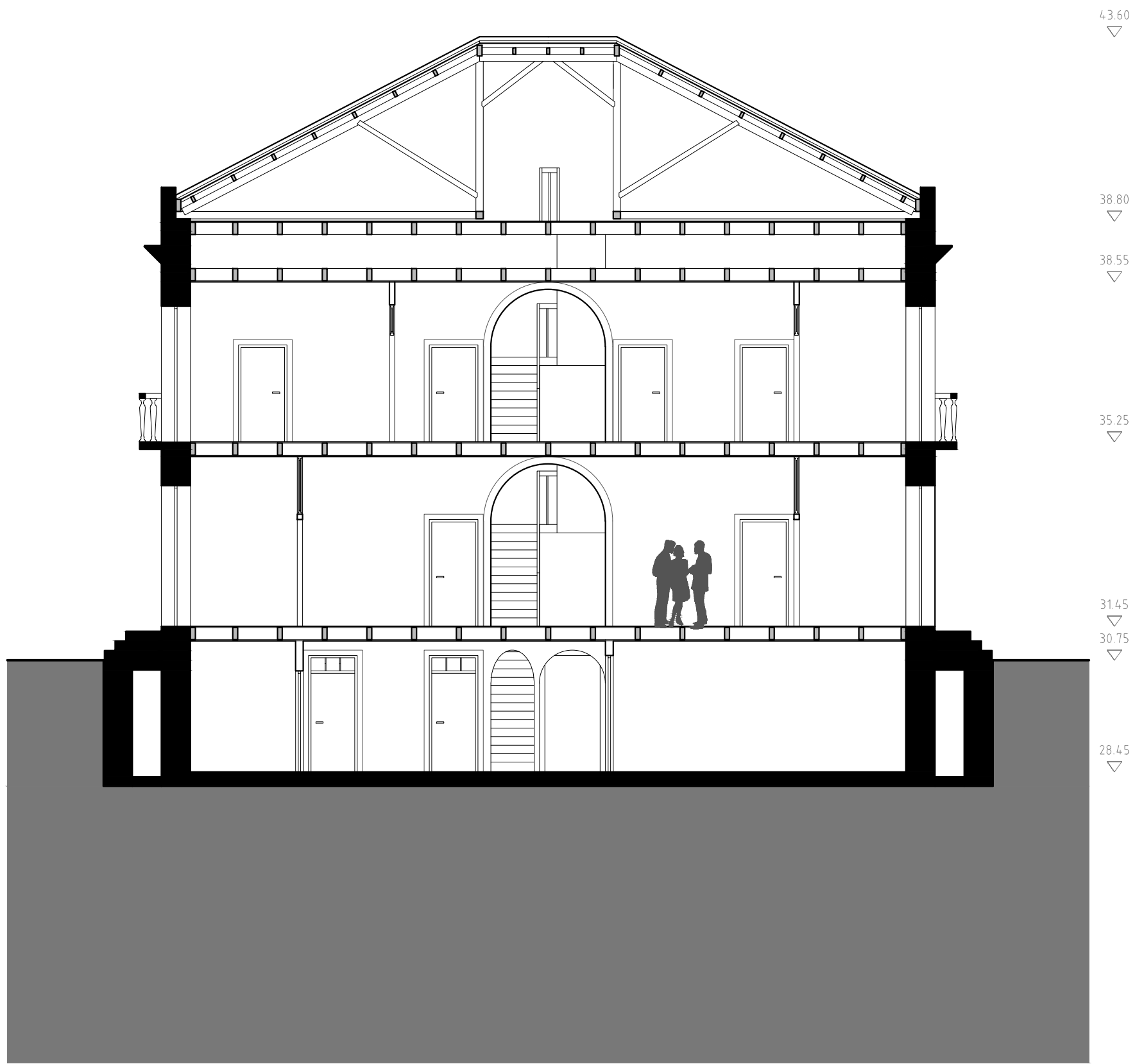
CORTE EE'
