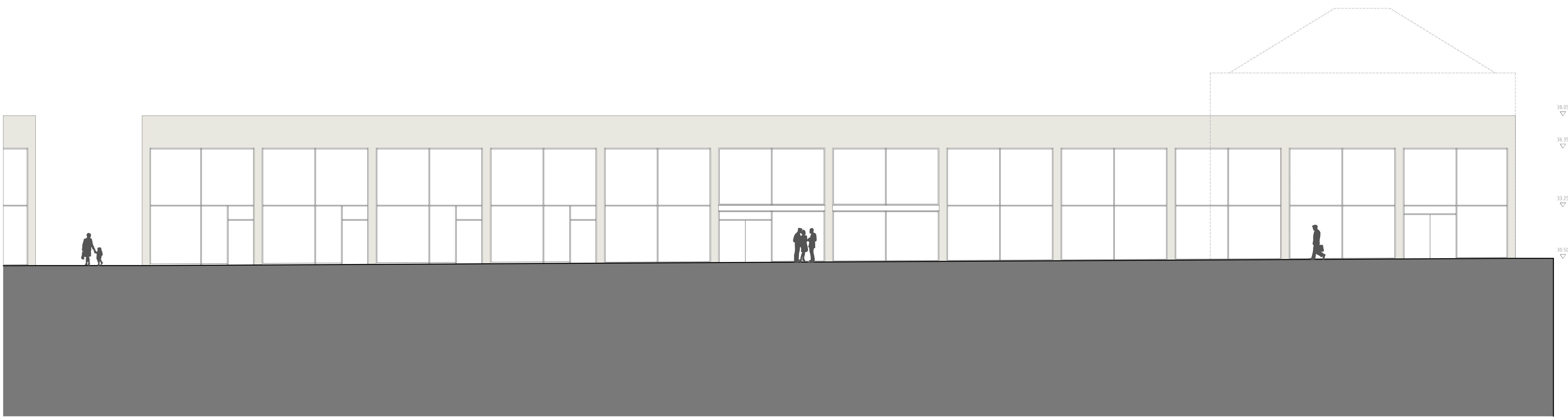
ALÇADO ESTE
