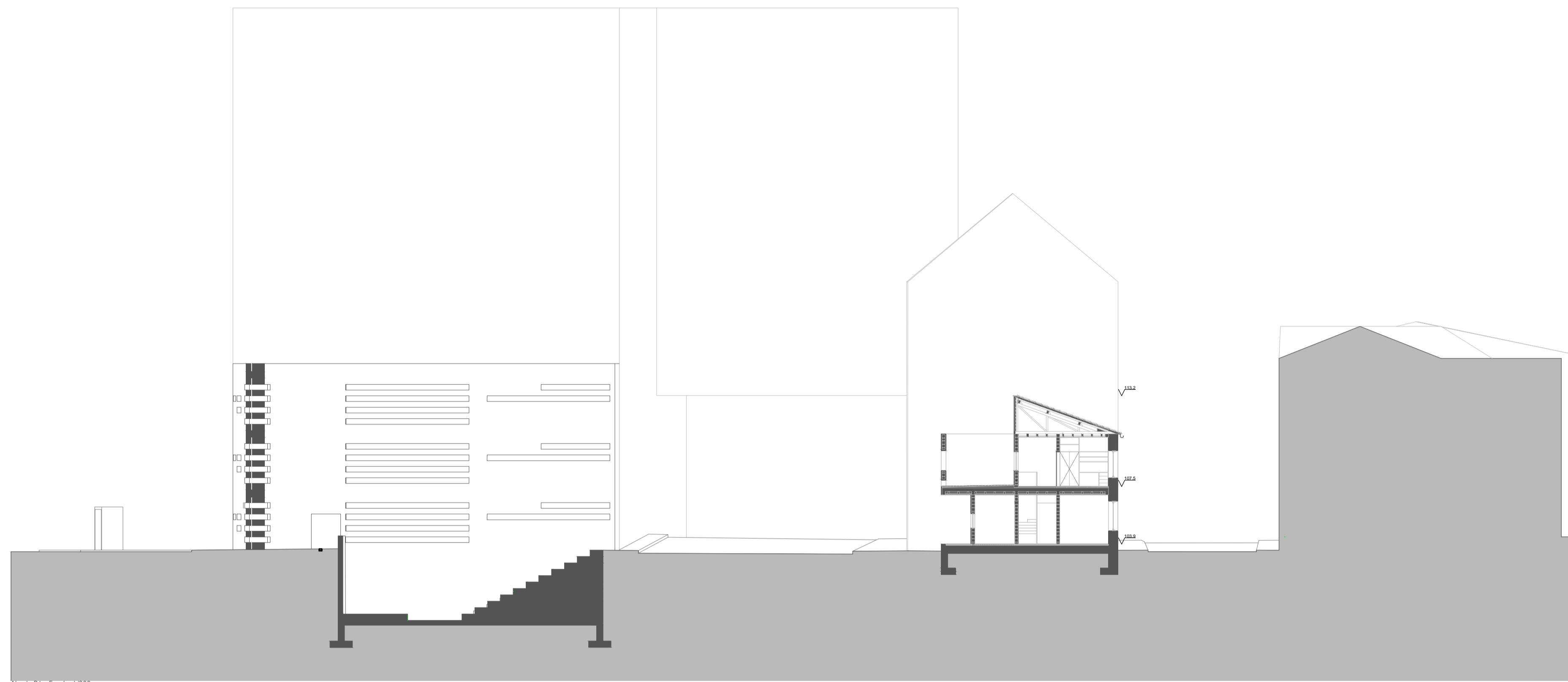
Alzado B1 - Escala: 1/200
