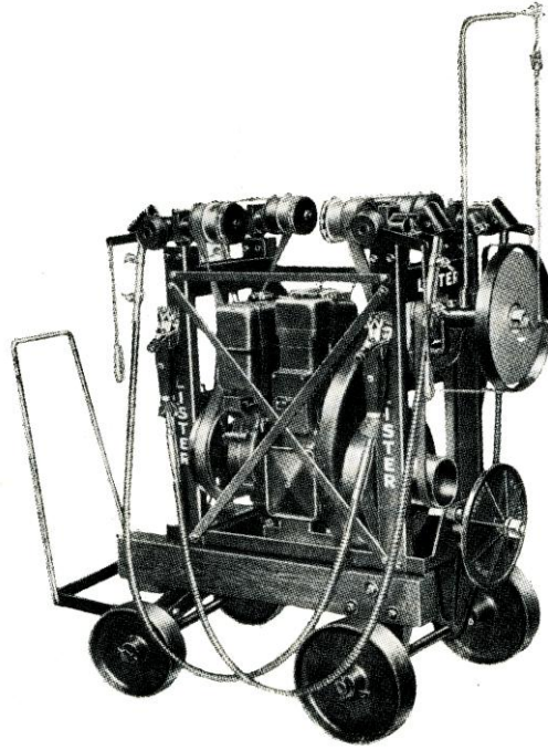
Fig. 38 – Gravura de uma Tosquiadeira mecânica. (Cartilha de Tosquia Mecânica, Junta Nacional dos Produtos Pecuários, Ministério da Economia – Secretaria de Estado do Comércio, p. 46)
