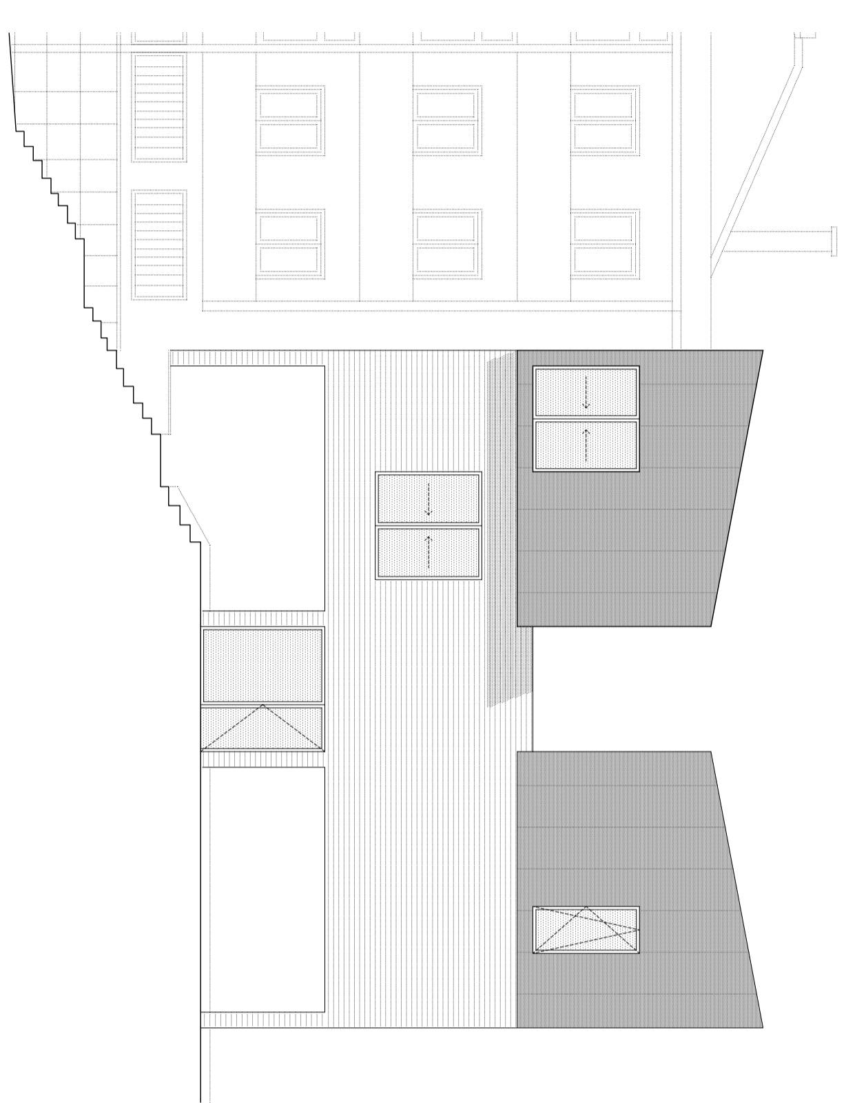
Alcáido Sur escala 1/100
