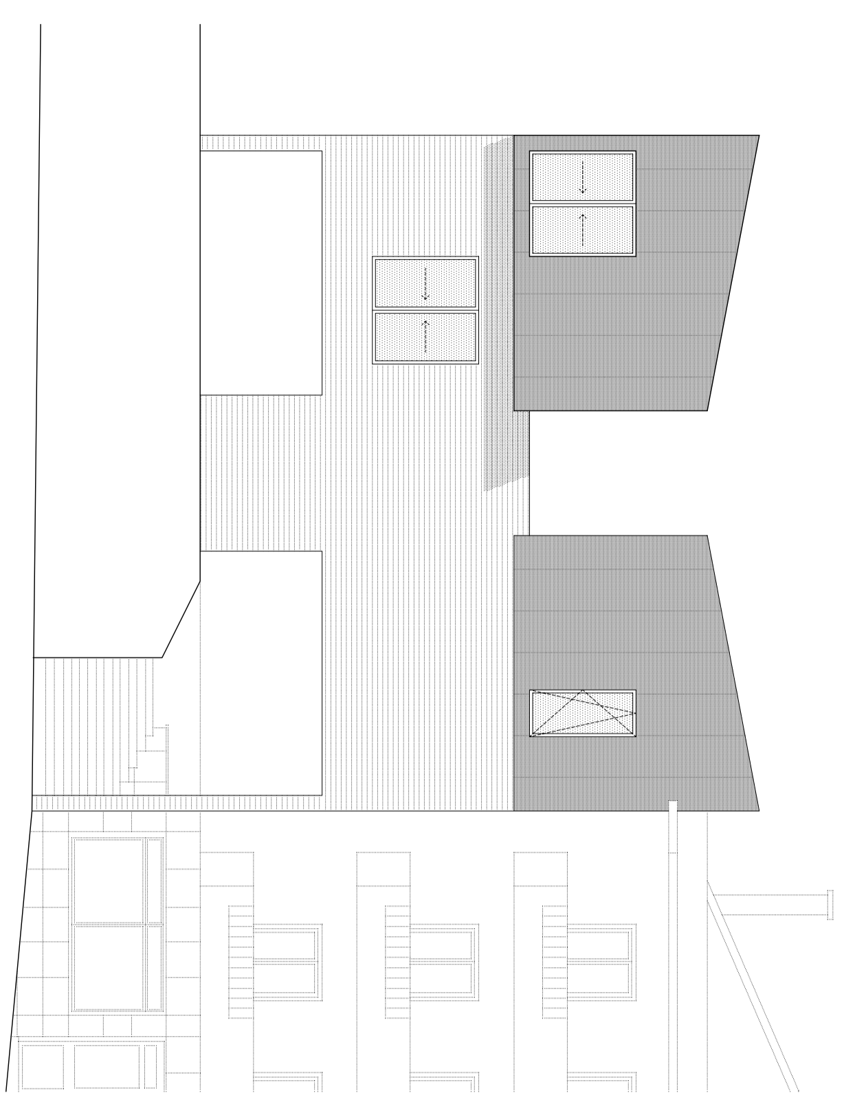
Alcáido Norte escala 1/100
