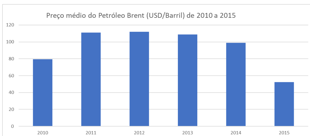
Figura 3.3 – Gráfico do Preço Médio do Petróleo Brent (USD/Barril) de 2010 a 2015
