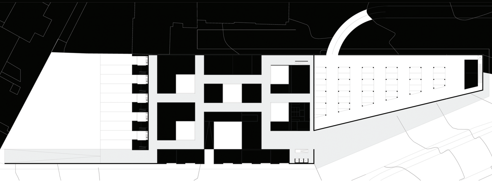
Planta do Piso Térreo ⊖ (sem escala)
