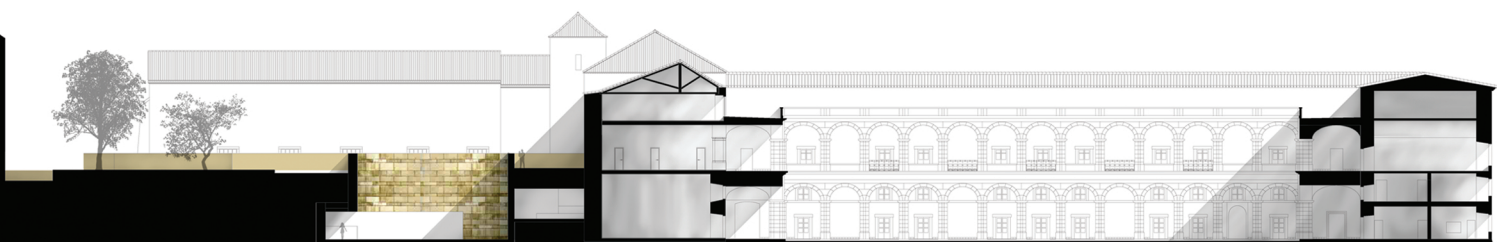
Corte pelo claustro do Convento (sem escala)
