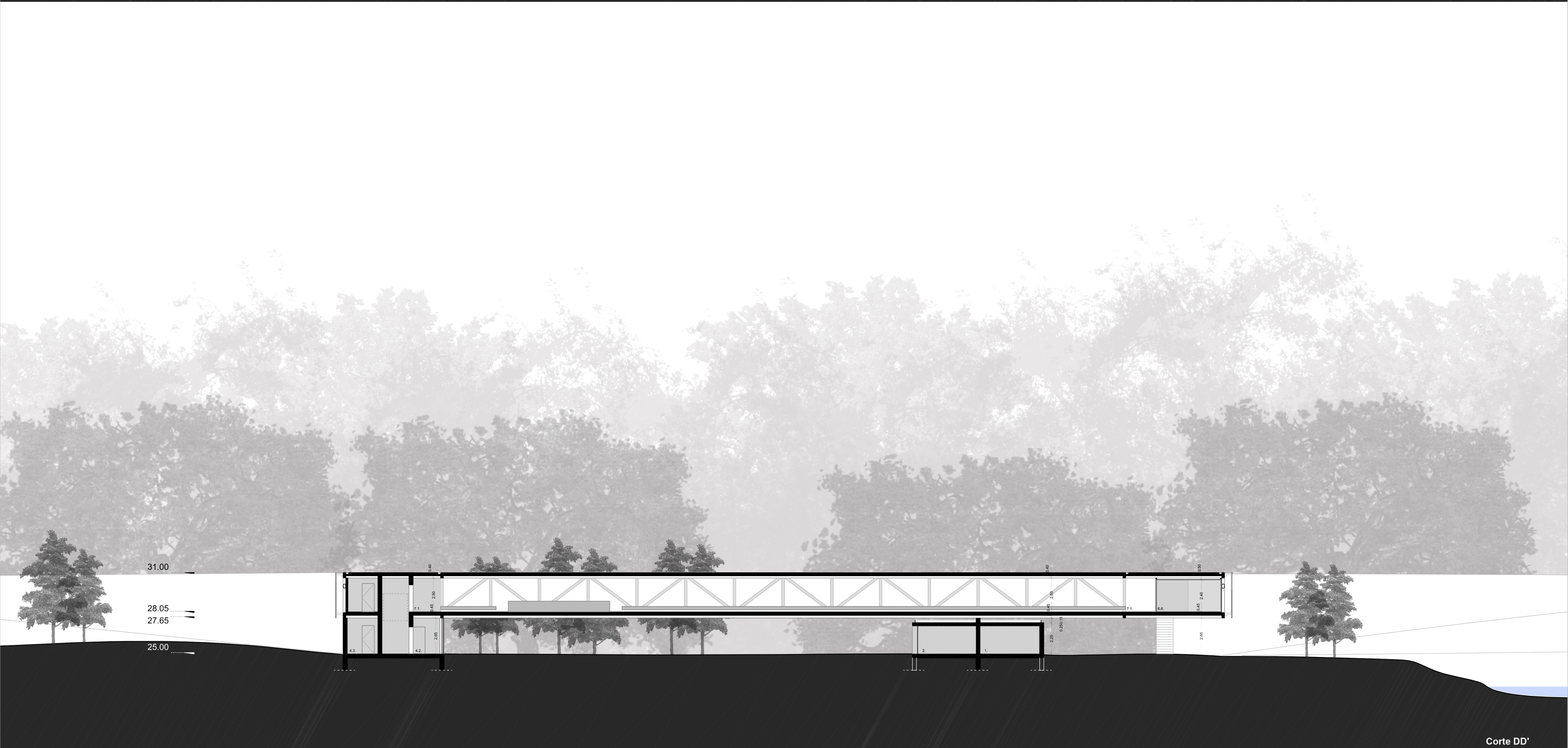
Corte DD'
