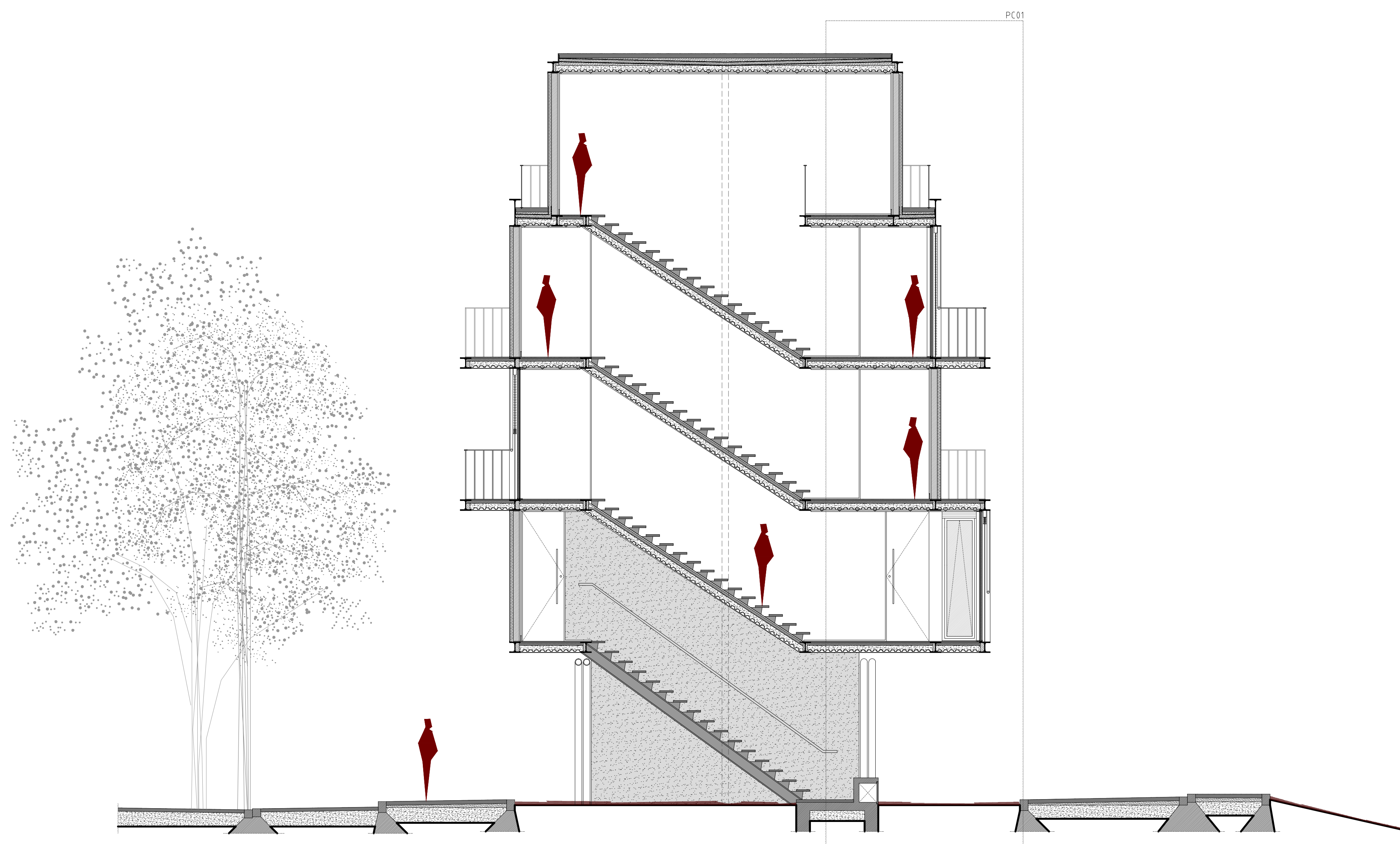
CORTE/ALÇADO DD
